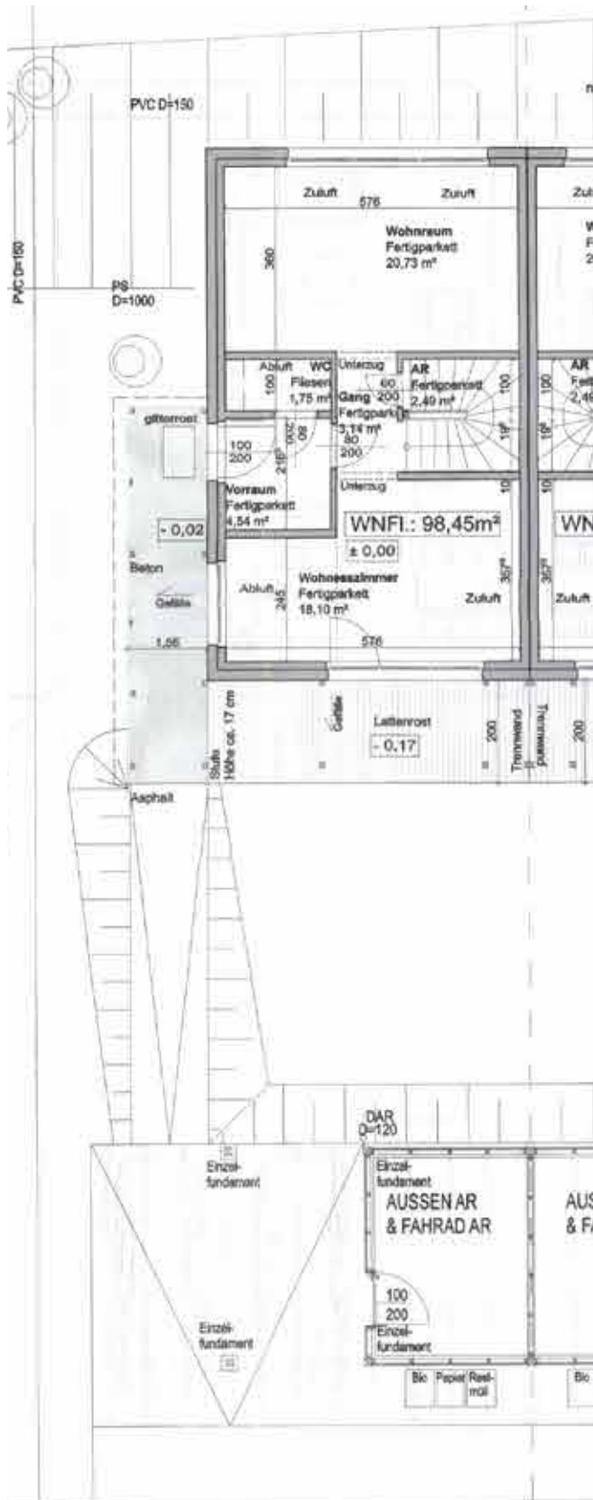
ERDGESCHOSS
